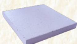
ref. 925.01 25x25x3 LAR REFRACTÁRIO BRANCO PRENSADO
